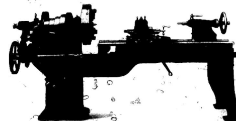
Leitspindel-Drehbank zum selbsttätigen Lang- und Handrohren und Gewindeschneiden (Dresdner AG, Dresden)
